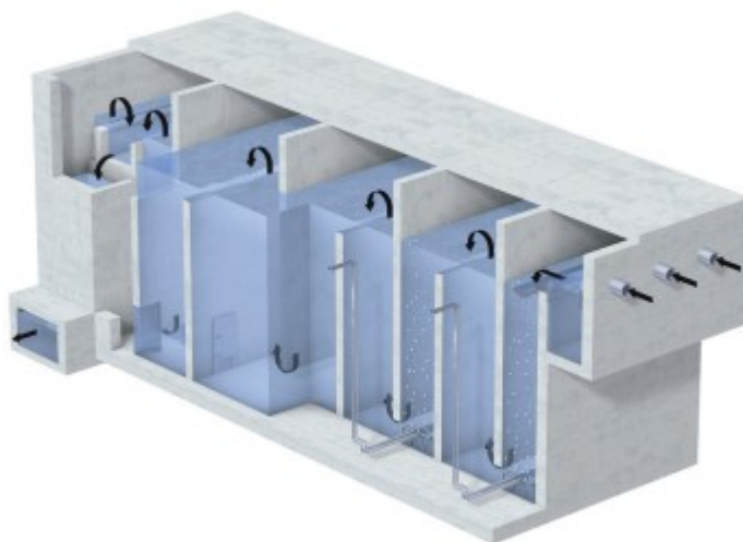
Abbildung 1: Ozonreaktor des Klärwerks Werdhölzli. Auf der Anlage sind vier solchen Reaktoren vorhanden. (Foto: Broschüre Klärwerk Werdhölzli)
