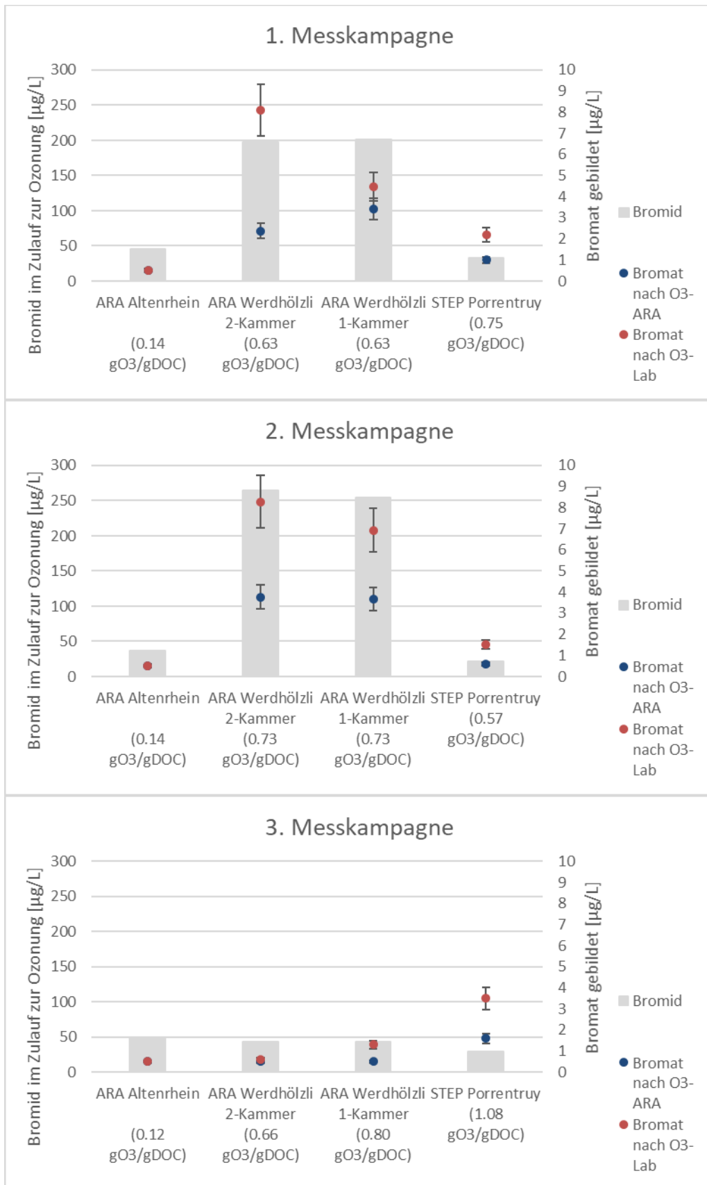
Abbildung 4: Bromid- und Bromat-Analysen für die drei unterschiedlichen Messkampagnen auf den drei Abwasserreinigungsanlagen. Die Messunsicherheit der Bromat-Messung beträgt ca. 15%.
