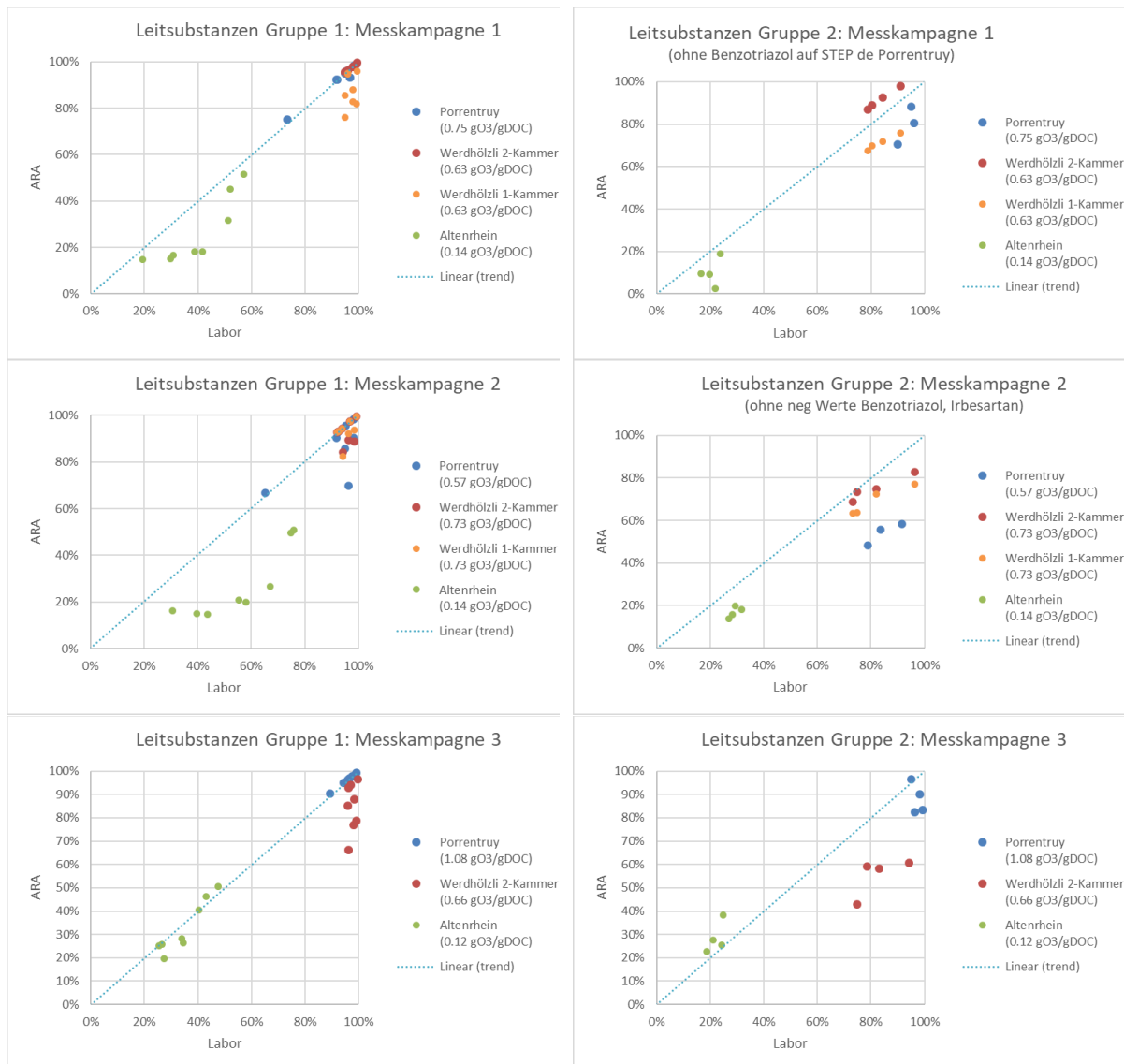
Abbildung 3: Berechnete Eliminationsleistungen der Leitsubstanzen (MV) nach der Ozonung im Labor und jeweils von den drei Kläranlagen für die drei unterschiedlichen Probenahmen.
