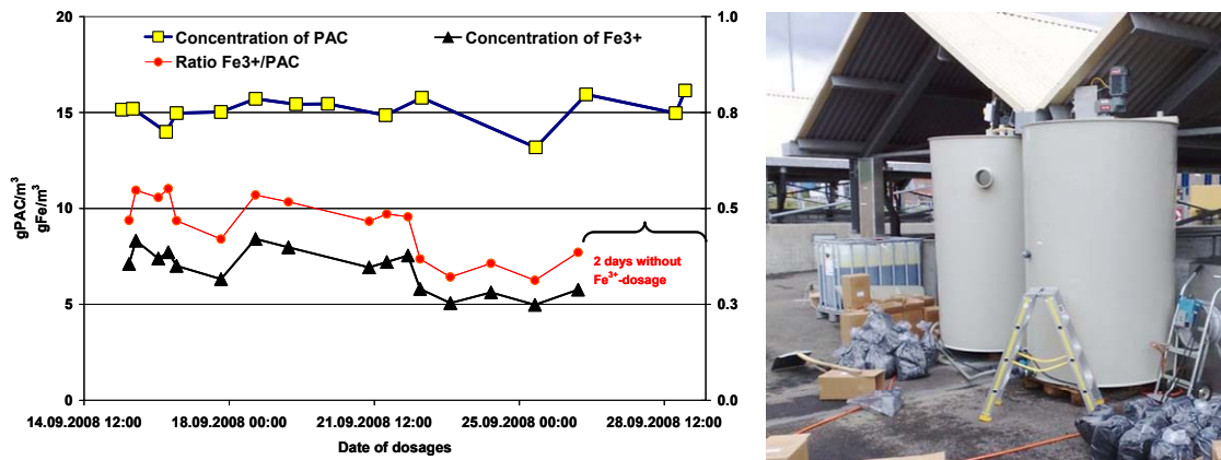
Abbildung 6A/B Tatsächliche Dosierverhältnisse und -konzentrationen im Versuchszeitraum, rechts Dosiereinrichtungen für Fällmittel und PAK-Suspension
